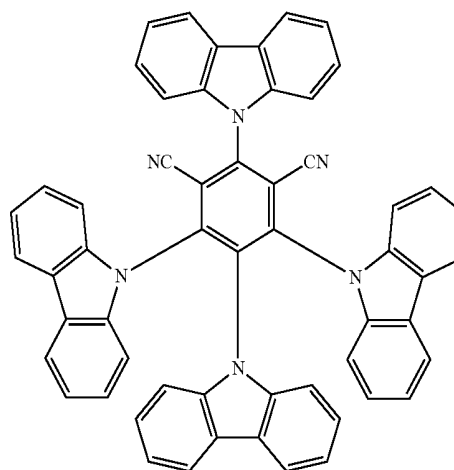
(4CzIPN)
