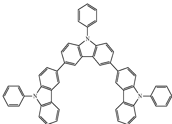
(Tris-PCz)
